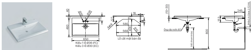
AL-2397V (EC/FC) | L-2397V (EC/FC)
