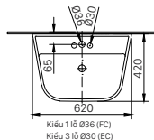
L-297V (EC/FC) | L-297VC (CHÂN CHẬU)
