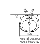
L-284V (EC/FC) | L-284VD (CHÂN CHẬU)
