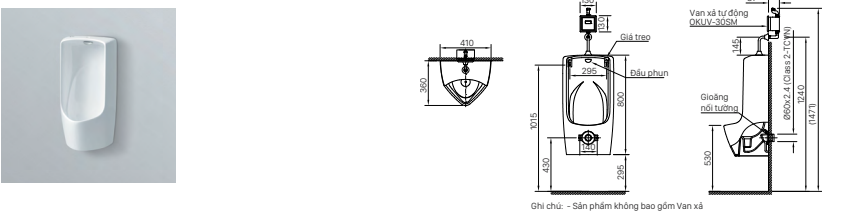
AU-411V | U-411V (VAN XẢ TỰ ĐỘNG OKUV-30SM)
