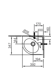
L-284V (EC/FC) | L-284VC(CHÂN CHẬU)
