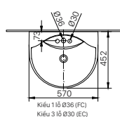
L-288V (EC/FC) | L-288VC (CHÂN CHẬU)
