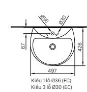
L-285V (EC/FC) | L-288VC (CHÂN CHẬU)
