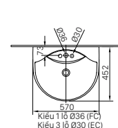
L-288V (EC/FC) | L-288VD (CHÂN CHẬU)
