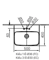
L-288V (EC/FC) | L-288VC (CHÂN CHẬU)
